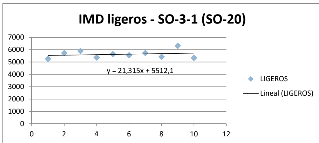
Imagen 8. Gráfico evolución IMD ligeros estación SO-3-1 (SO-20)
