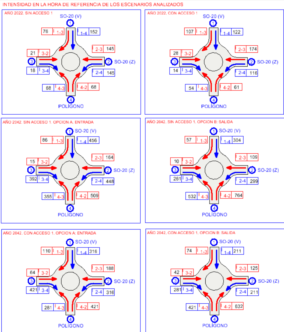
Imagen 21. Esquema Valores Intensidad Hora de referencia
