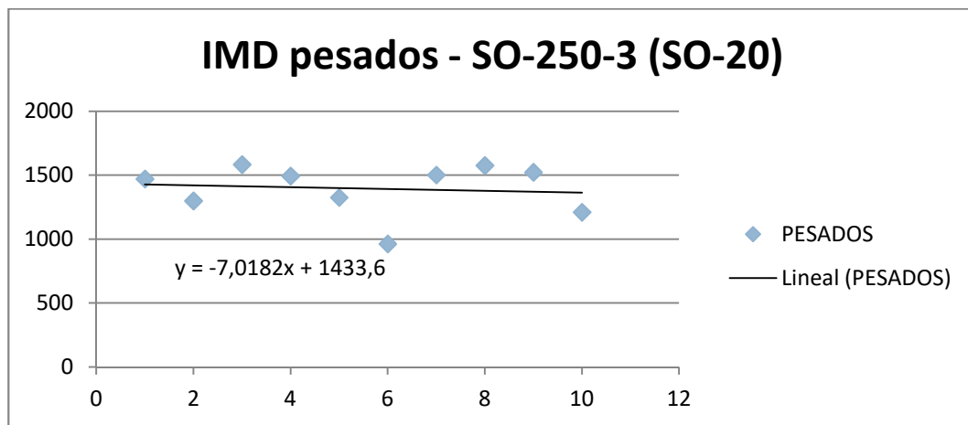
Imagen 12.- Evolución IMD pesados. Estación SO-250-3 (SO-20)
