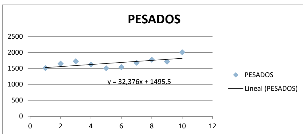
Imagen 9. Gráfico evolución IMD pesados estación SO-3-1 (SO-20)
