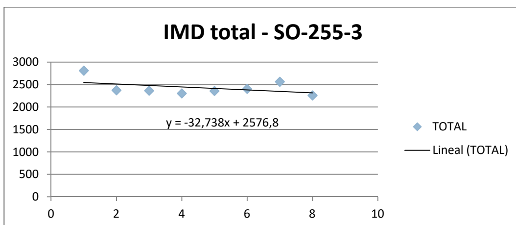
Imagen 4. Evolución IMD estación SO-255-3 (N-234)
