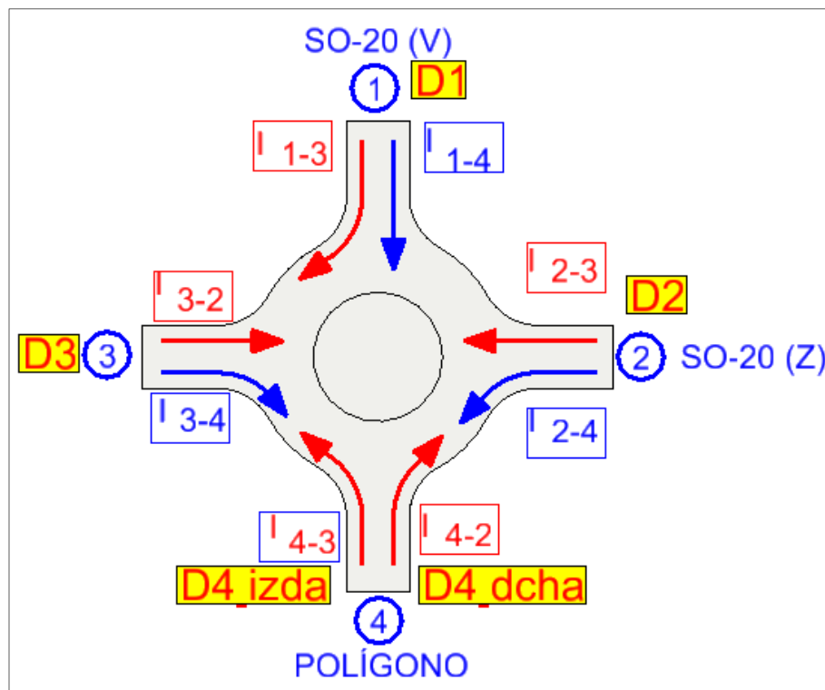
Imagen 25. Demandas en cada carril de entrada
