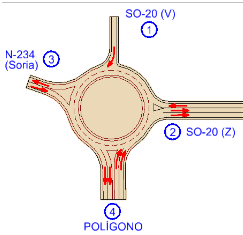
Imagen 15.- Configuración carriles en la glorieta
