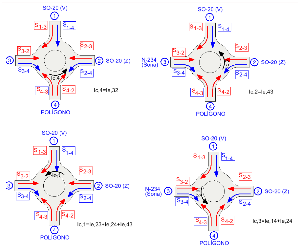
Imagen 24. Intensidad prioritaria en conflicto en cada pata
