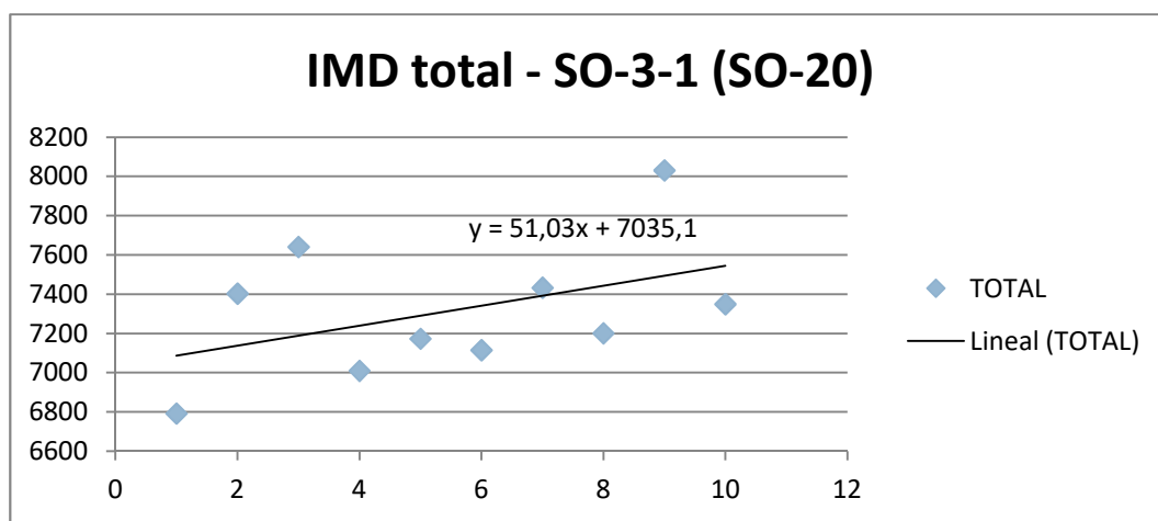
Imagen 7. Gráfico evolución IMD estación SO-3-1 (SO-20)
