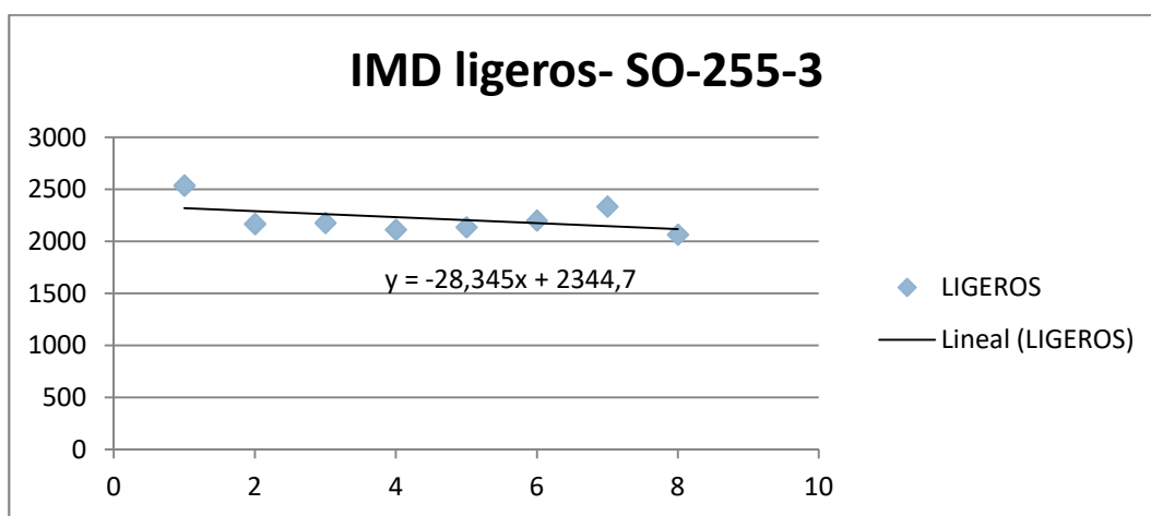
Imagen 5.-Evolución IMD ligeros estación SO-255-3 (N-234)
