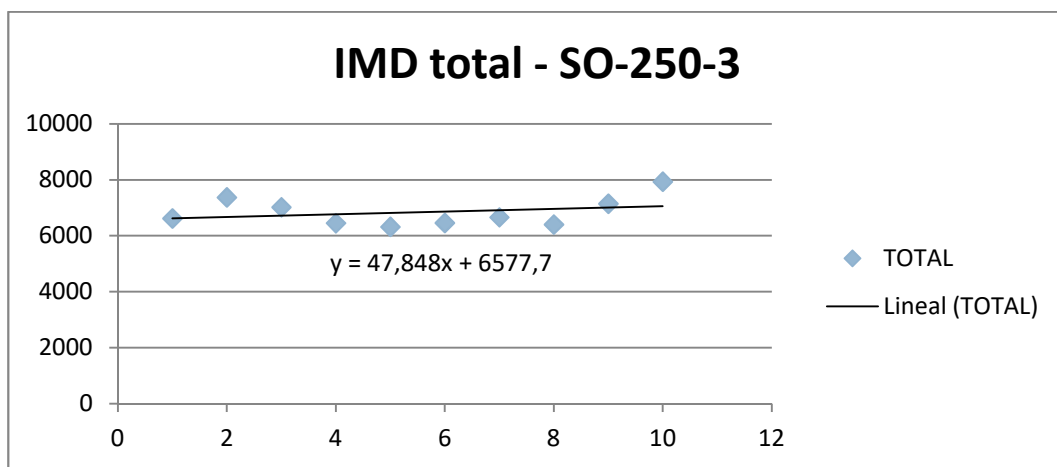
Imagen 10. Evolución IMD total. Estación SO-250-3
