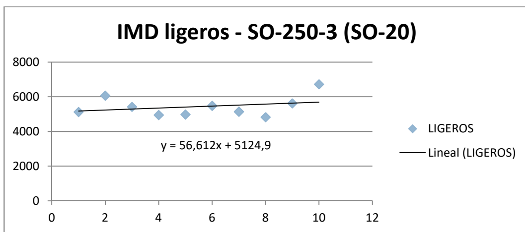
Imagen 11. Evolución IMD ligeros. Estación SO-250-3 (SO-20)
