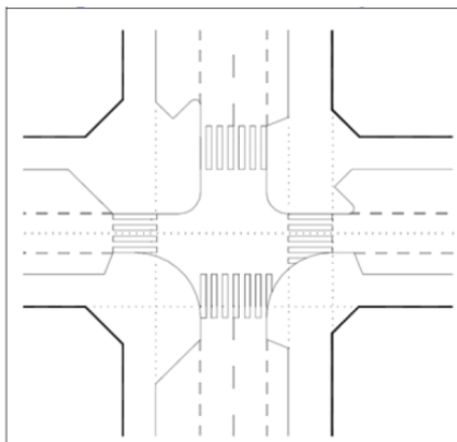
Diseño de orejas en intersección
